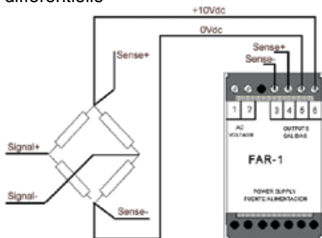
Alimentation FAR-1 avec cellule de charge
